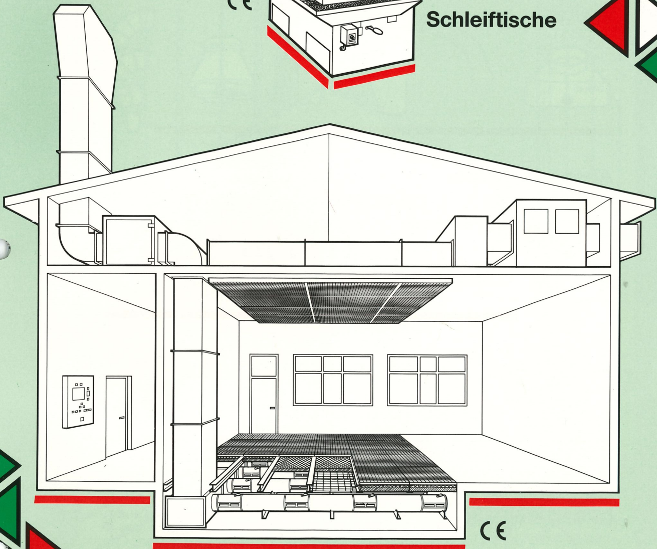
Underfloor Absaugsystem für Lackerräume
